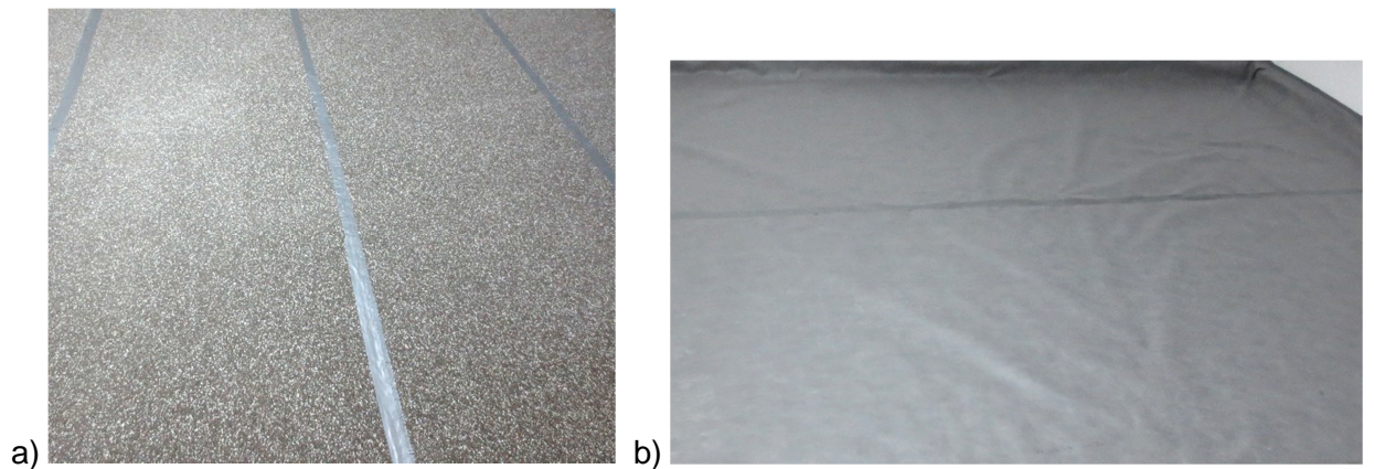
Abbildung A 2.1: Montagesituation – Einbau der Ausgleichs- und Schalldämmschüttung
